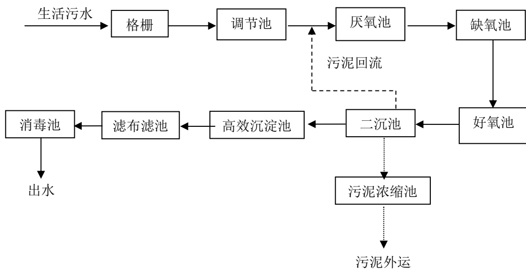
图 2.2-2 戴庄镇污水处理厂工艺流程及产污环节图
