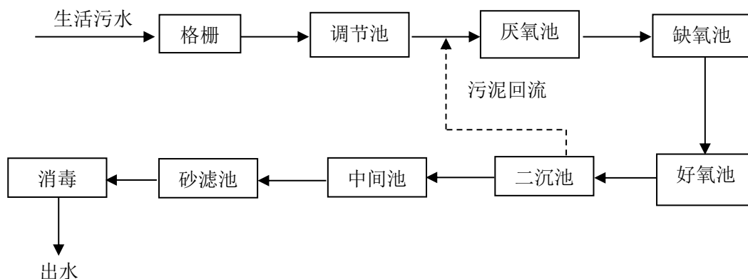
图 2.2-2 土山镇污水处理厂一期工艺流程及产污环节图
